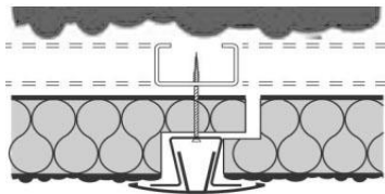
onregelmatige muur of plafond (metaal gril of CLS hout)
