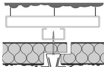
hangend plafond (metaal gril)
